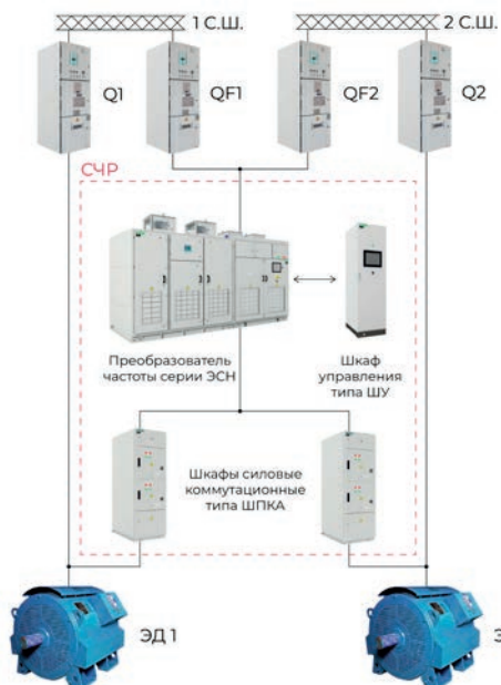
г) Многодвигательный вариант с использованием одного ПЧ
