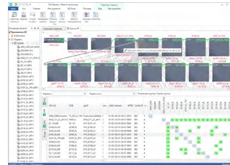
Привязки GOOSE-сообщений
