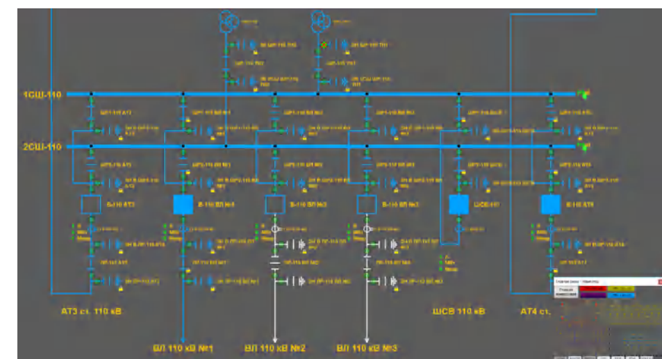
Подробные схемы распределителей РУ (ОРУ, КРУ, ЗРУ и т. д.)
